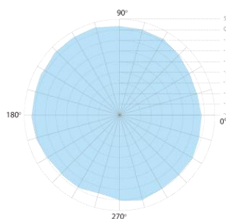
2.4GHz 2D 無線場形@ 垂直方向
