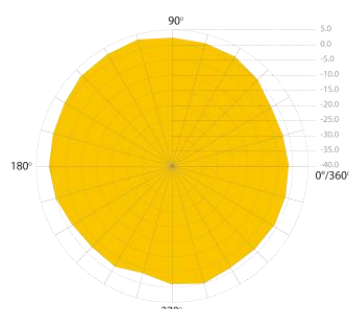
5GHz 2D 無線場形@ 水平方向
