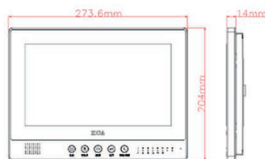
尺寸圖
