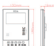
尺寸圖
