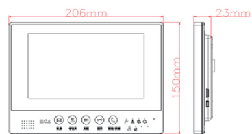
尺寸圖
