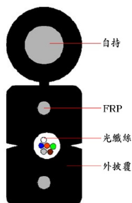
示意圖
